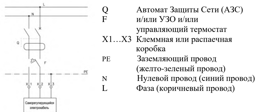
Рис. 2. Схема подключения электрообогрева кровельной воронки HL64.1BH к электрической сети.
