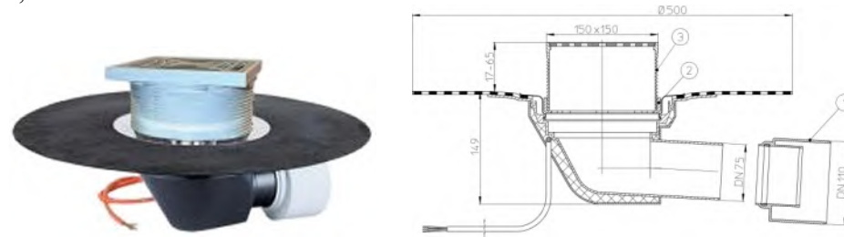
Рис. 1. Кровельная воронка с электрообогревом HL64.1BH
